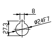
INPUT SHAFT
